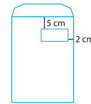
Code 1920 ● Formaat 22,9 x 32,4 cm met venster 5 x 11 cm.
